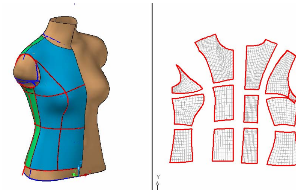
Пробная версия основы прилегающего блузона с разделением на детали и развертками.
